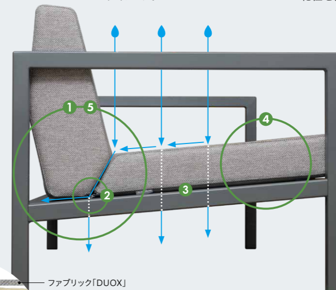
1 水をためないクロスカット カビや汚れを防止するために水がたまりやすいコーナーはクロスカットに。
